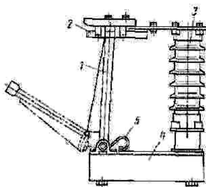
Рис. 6. Короткозамыкатель КЗ-35:
