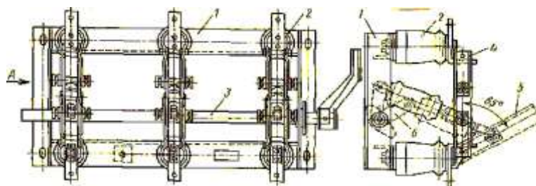
Рис. 5 Трехполюсный разъединитель
